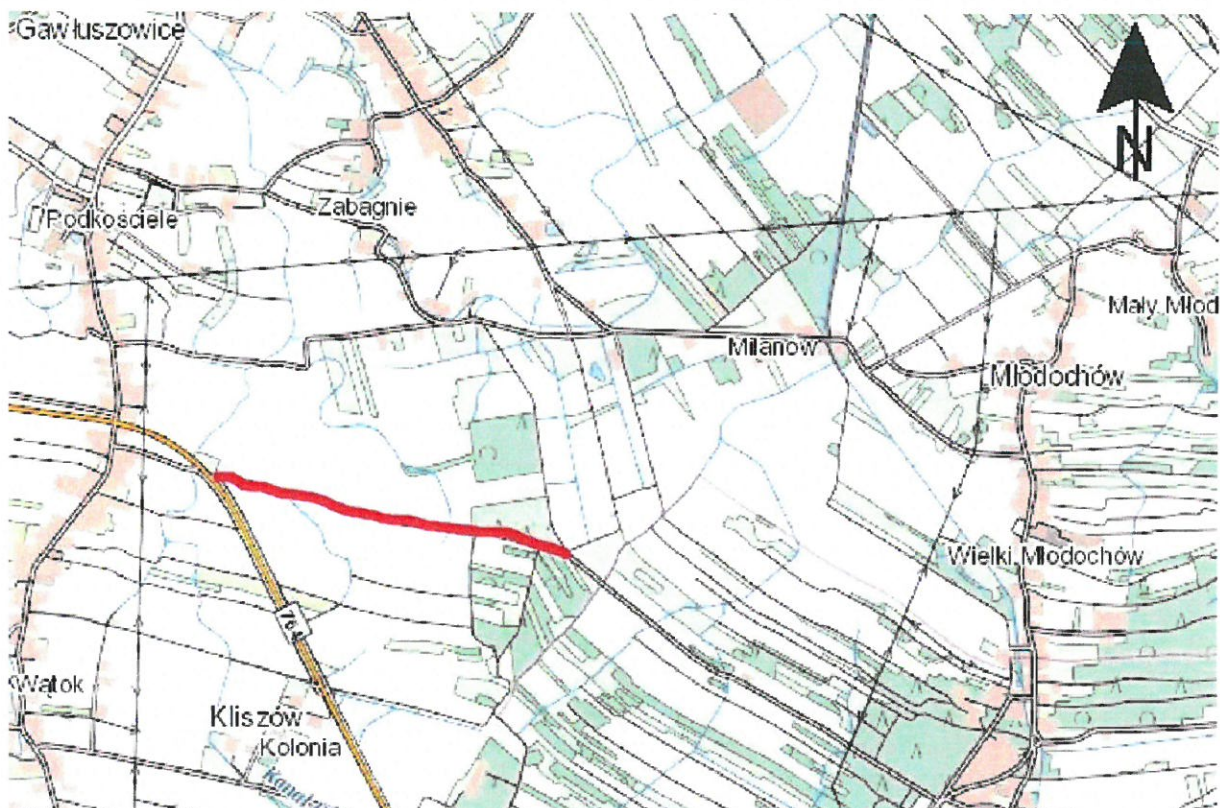
Rysunek 8 Odcinek drogi Kliszów - Borki przewidziany do modernizacji.
